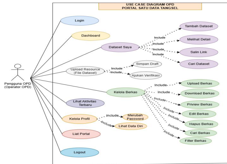
Gambar.A. Use Case Diagram Pengguna OPD
