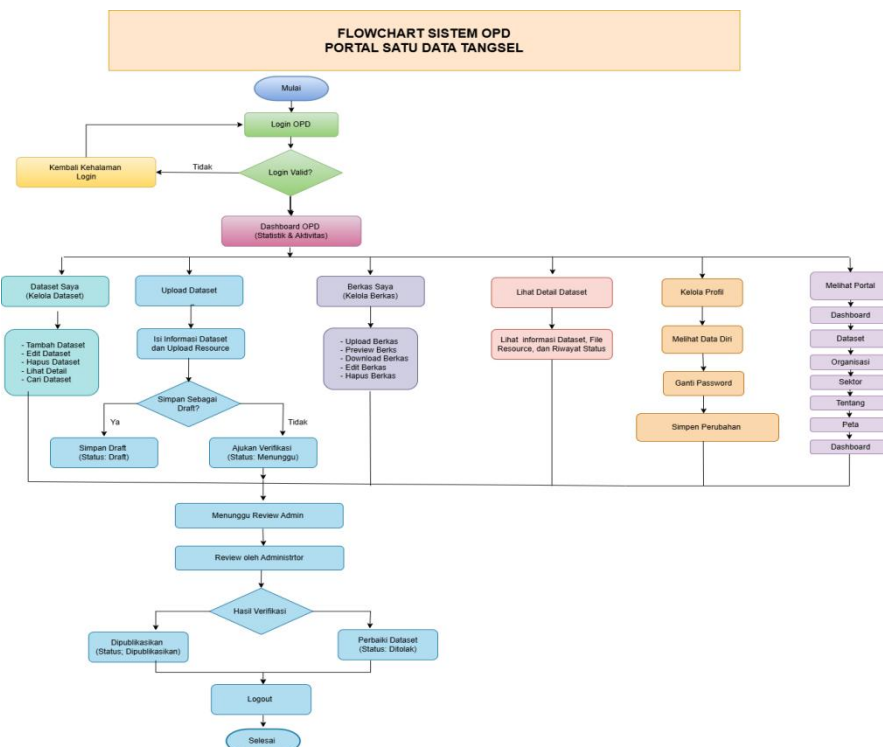
Gambar.B. Flowchart Diagram Pengguna OPD
