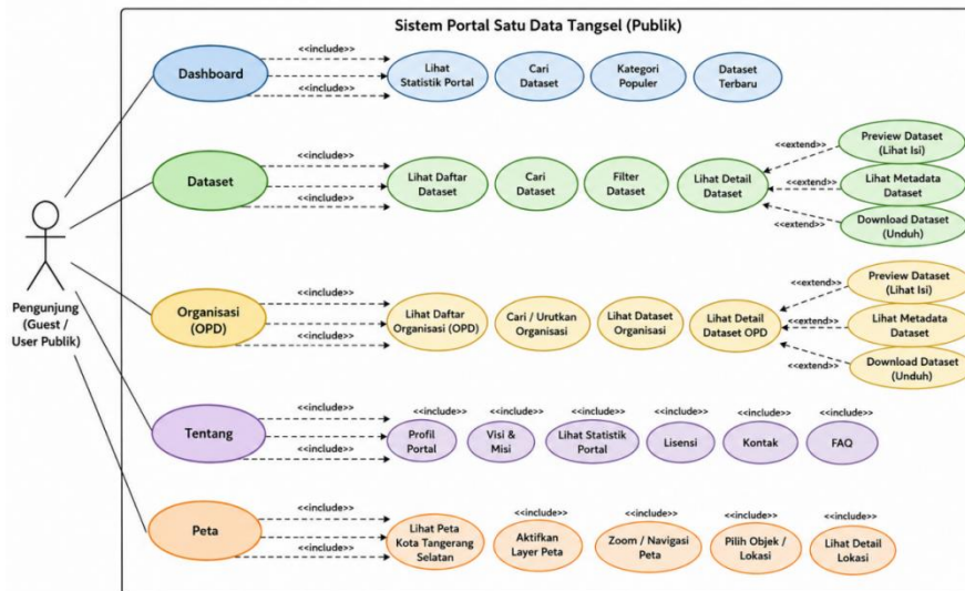
Gambar.C. Use Case Diagram Pengguna Publik
